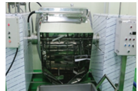
가열 교반기
